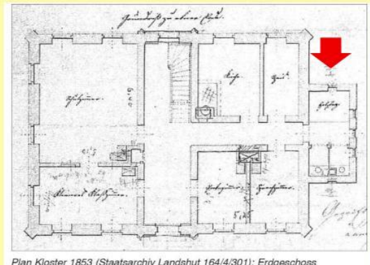
Plan Kloster 1853 (Staatsarchiv Landshut 164/4/301): Erdgeschoss
